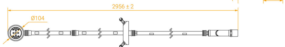
向上型細水霧噴頭及三根延長管
