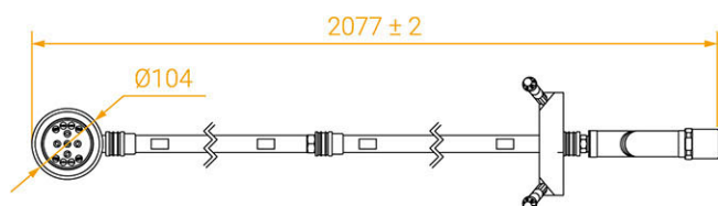
向上型細水霧噴頭及三根延長管
