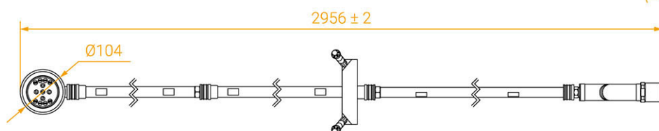
向上型細水霧噴頭及三根延長管
